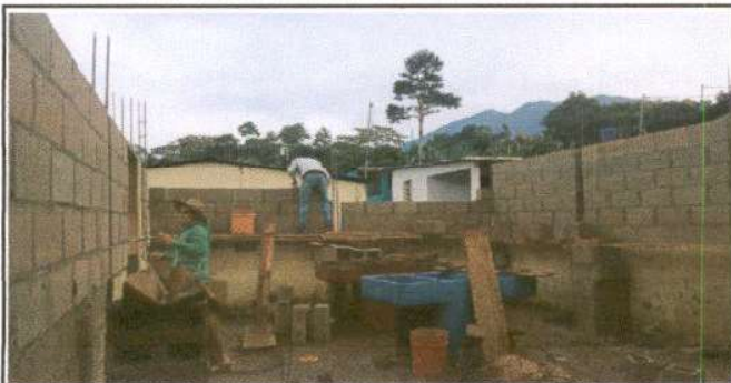
Foto 1: Sustitución de lámina por lámina troquelada aluzinc calibre 26, 63m2
